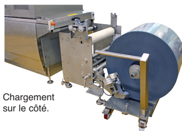
Faire rouler la bobine sur le chariot.
