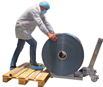
Faire rouler la bobine sur le chariot.
